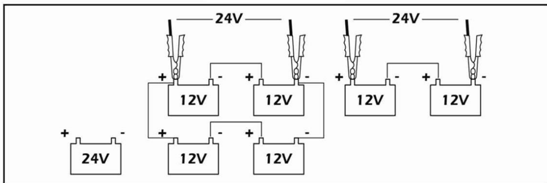
SCHEMAT 24V
